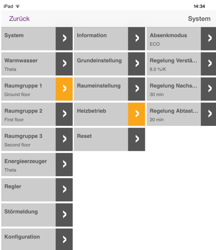
Abb. 8: Einstellung Raumregelung
