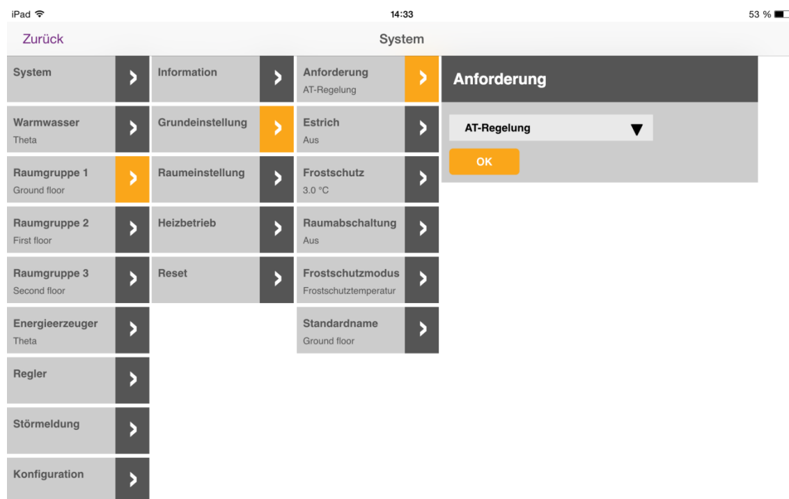
Abb. 7: Auswahl Anforderung
