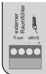
Anschlüsse MB 6x02 Ansicht Rückseite
