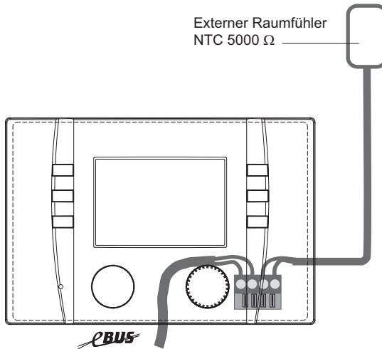
Anschlüsse MB 6x02 Ansicht Rückseite
