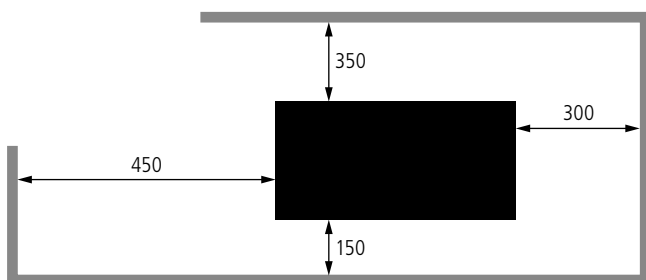
Abb. 5: Mindestabstände (Angaben in mm)
